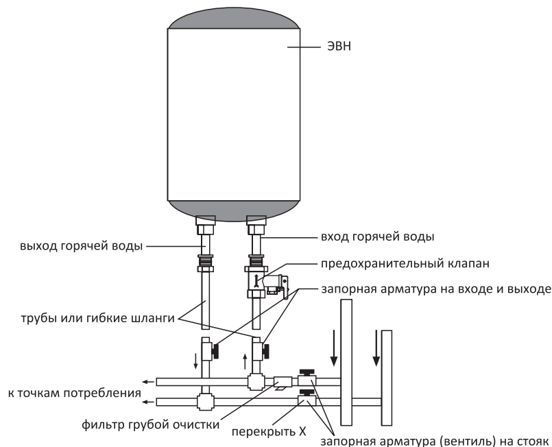
Гидравлическая система вертикальная настенная установка
