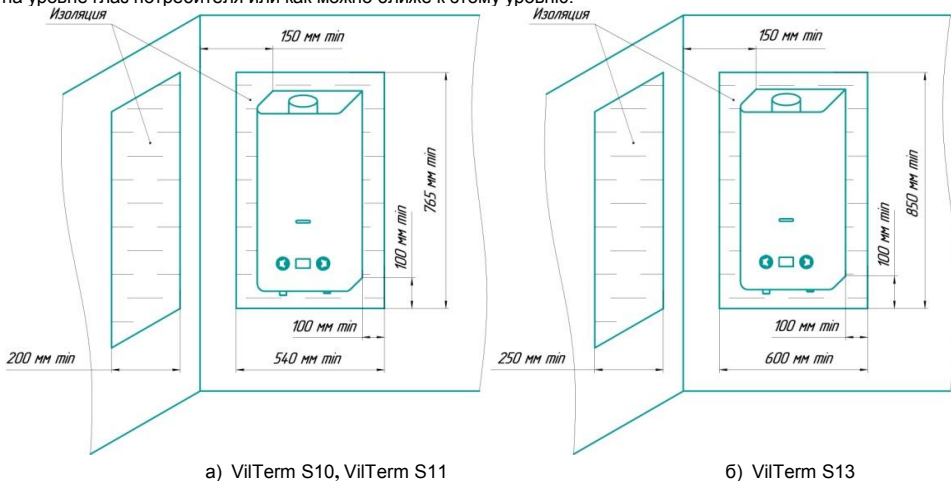
Рисунок 2. Пример установки аппаратов на трудносгораемых стенах
